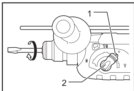
► 1. Bouton de verrouillage 2. Bouton de changement de mode
