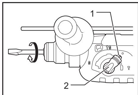
► 1. Botón de bloqueo 2. Perilla que cambia el modo de acción
